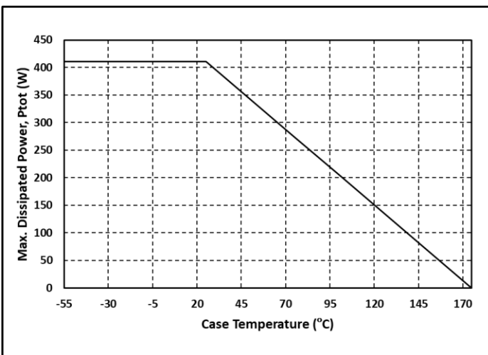
图. 24 最大功耗降额和温度关系曲线
