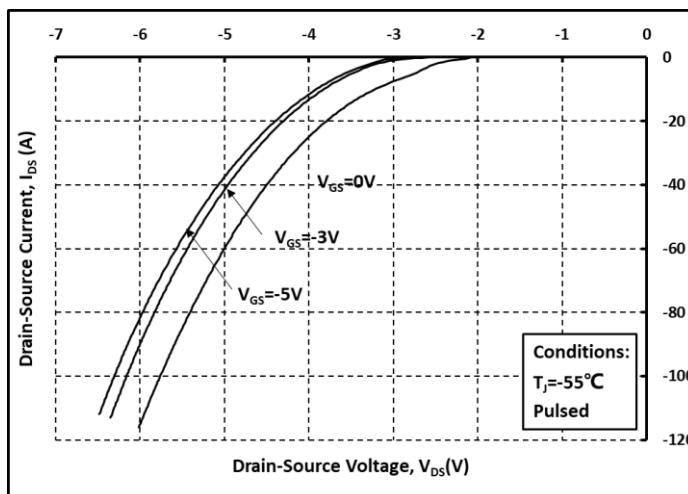
图. 10 体二极管导通曲线 @ T_j = -55^{\circ}C
